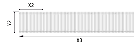
GP3 Dimensiones de las rejillas superiores
