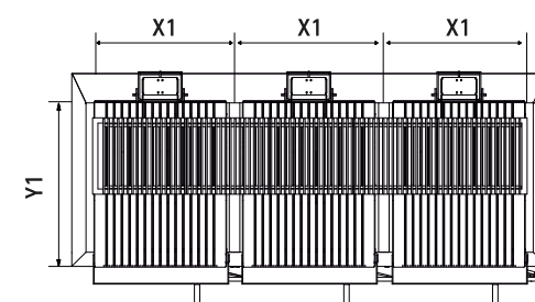
Dimensiones de las rejillas de la parrilla GP3
