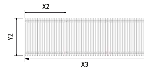
Dimensiones de las rejillas de la parrilla GP2
