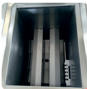
Detalle Cuba Tank Detail Détail de Cuve
